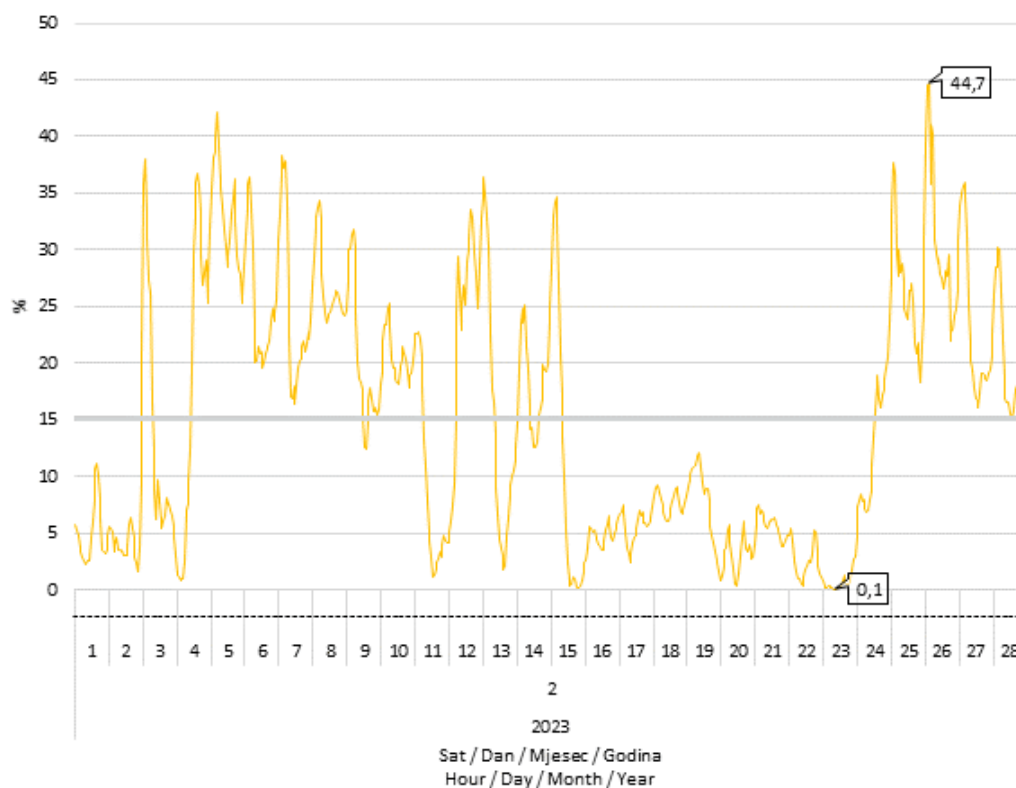
Slika 8 Udio proizvodnje vjetroelektrana u pokrivanju satnog opterećenja elektroenergetskog sustava u veljači 2023. godine
