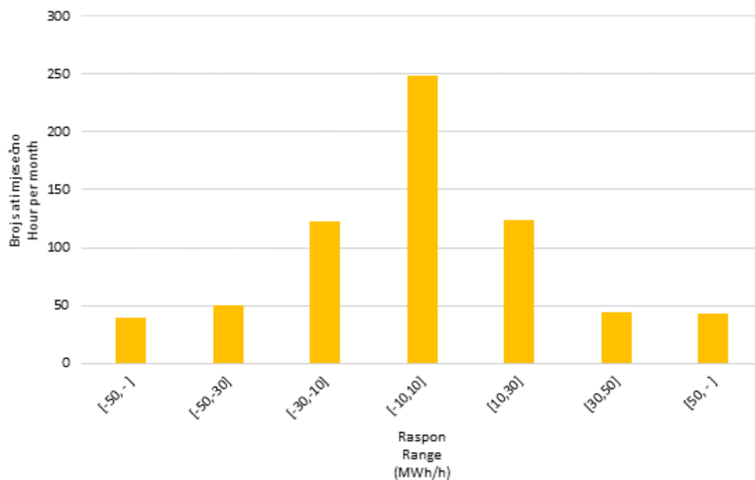
Slika 10 Statistička raspodjela satnih promjena proizvodnje VE u veljači 2023. godine
