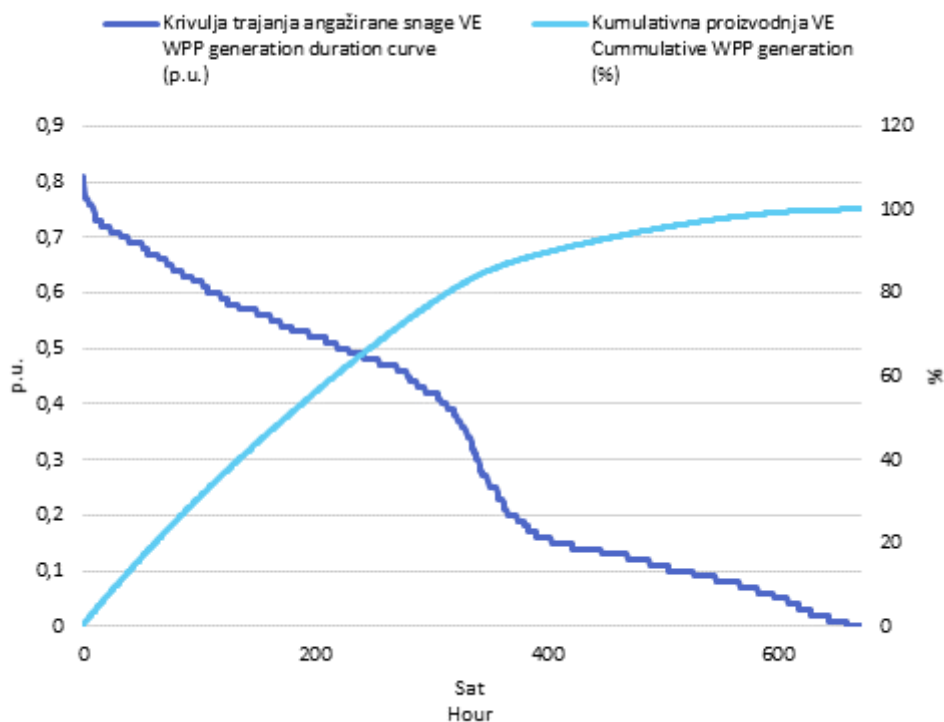
Slika 3 Krivulja trajanja angažirane snage svih VE i kumulativna proizvodnja VE u veljači 2023. godine u jediničnim vrijednostima
