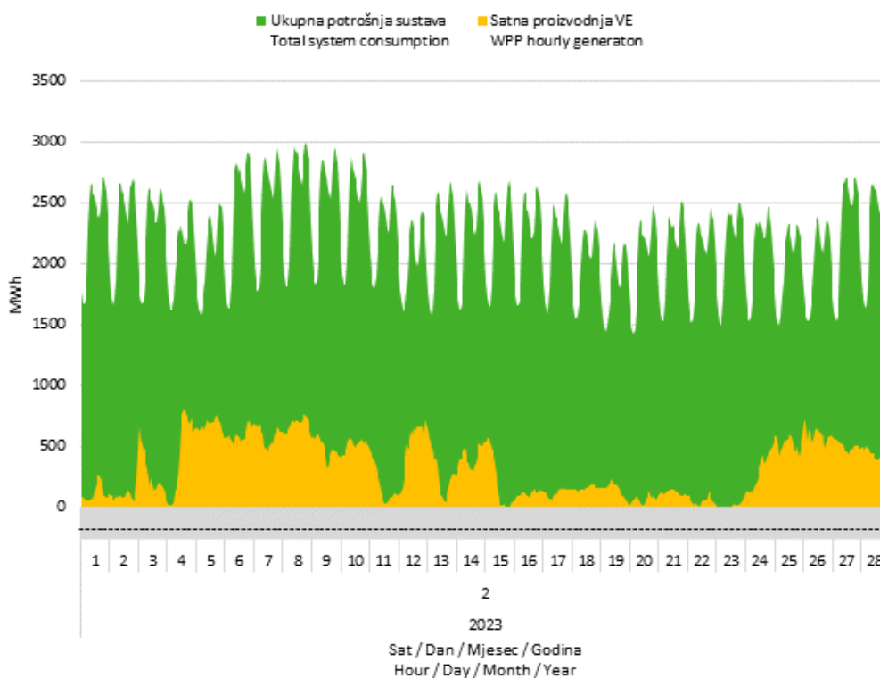
Slika 7 Usporedba satnog dijagrama opterećenja sustava i proizvodnje vjetroelektrana u veljači 2023. godine
