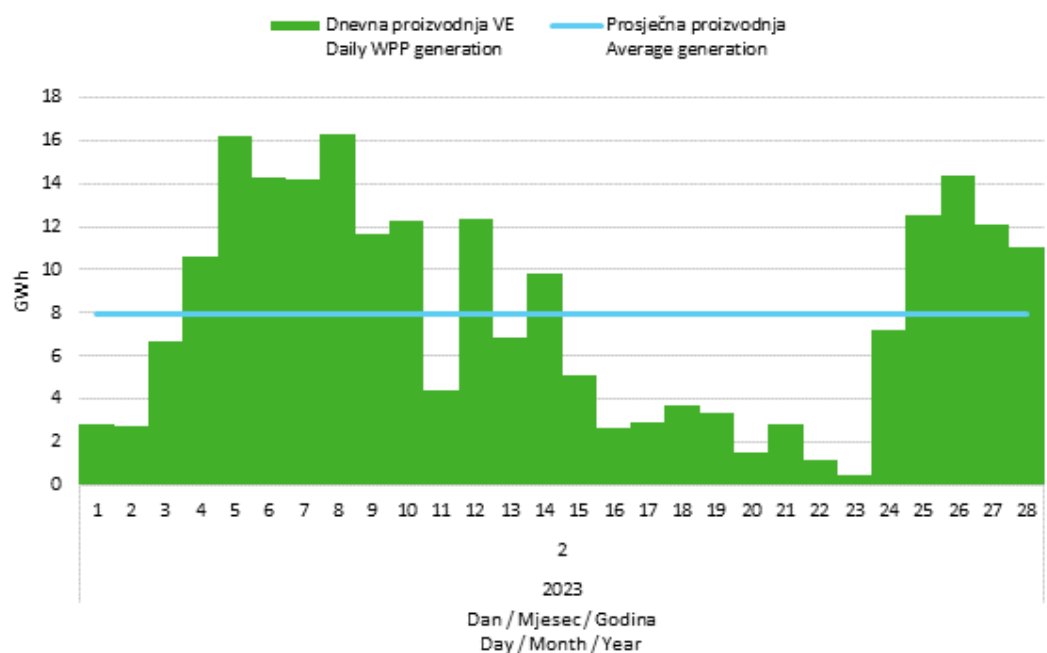
Slika 5 Dnevna proizvodnja svih vjetroelektrana u veljači 2023. godine
