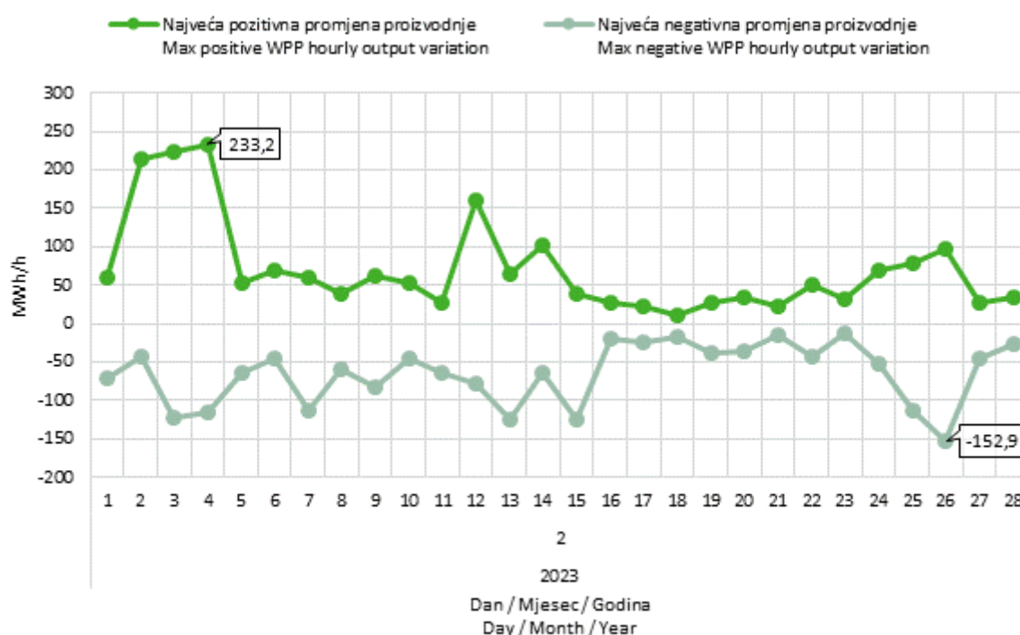
Slika 9 Maksimalna pozitivna i maksimalna negativna promjena satne proizvodnje VE u veljači 2023. godine
