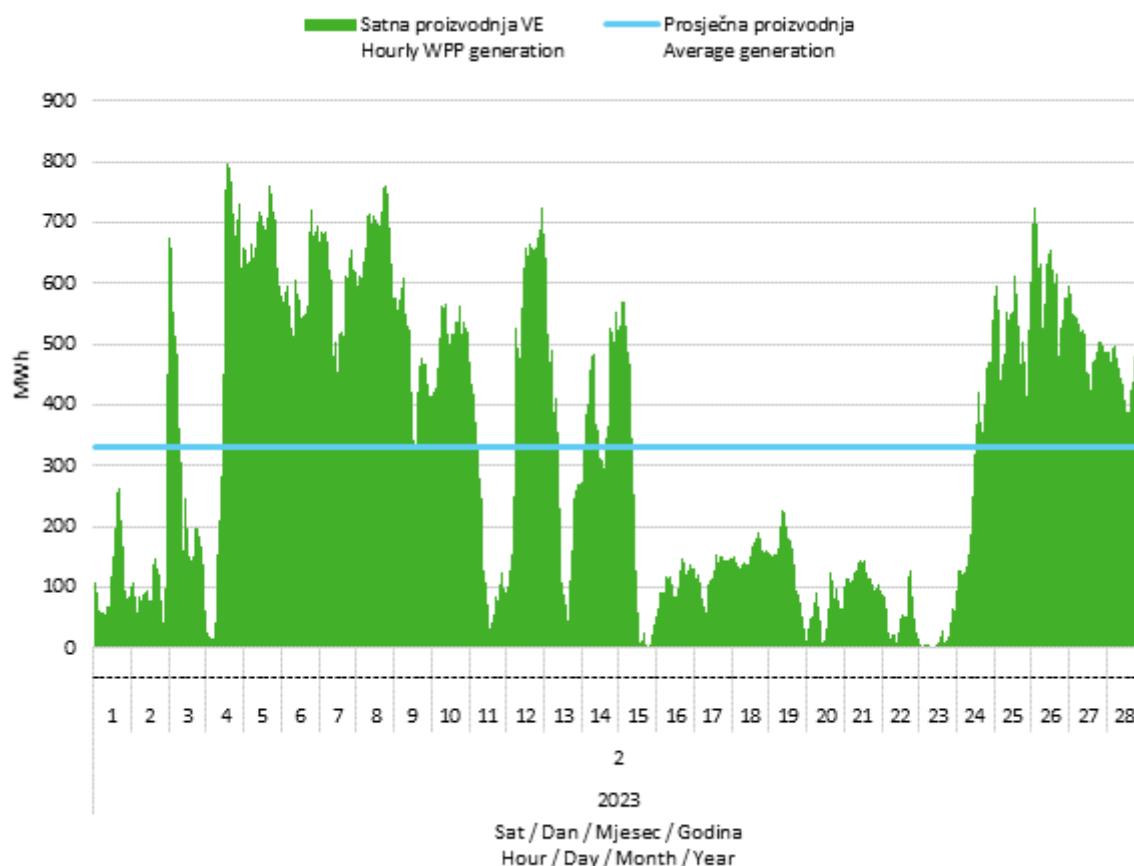
Slika 2 Satna proizvodnja svih vjetroelektrana u veljači 2023. godine
