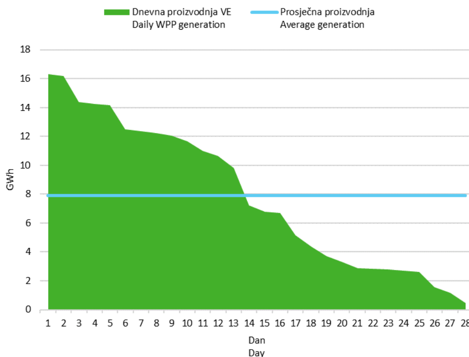
Slika 6 Krivulja trajanja dnevne proizvodnje vjetroelektrana u veljači 2023. godine
